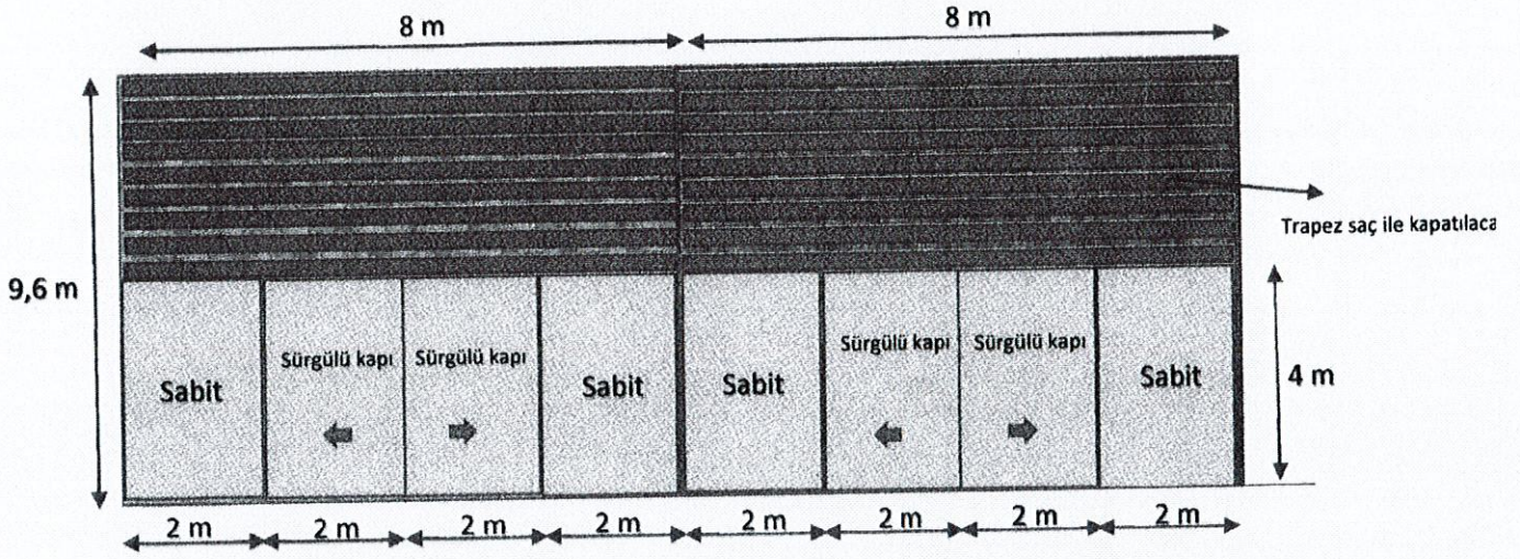
Çizim 3.2. Kapatılarak depo yapılacak olan kısımların ön görünüş resimleri
